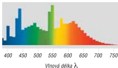
Spektrum denního světla zářivky BIOLUX®. Zařízení velmi rovnoměrně zahrnuje celý viditelný rozsah.
